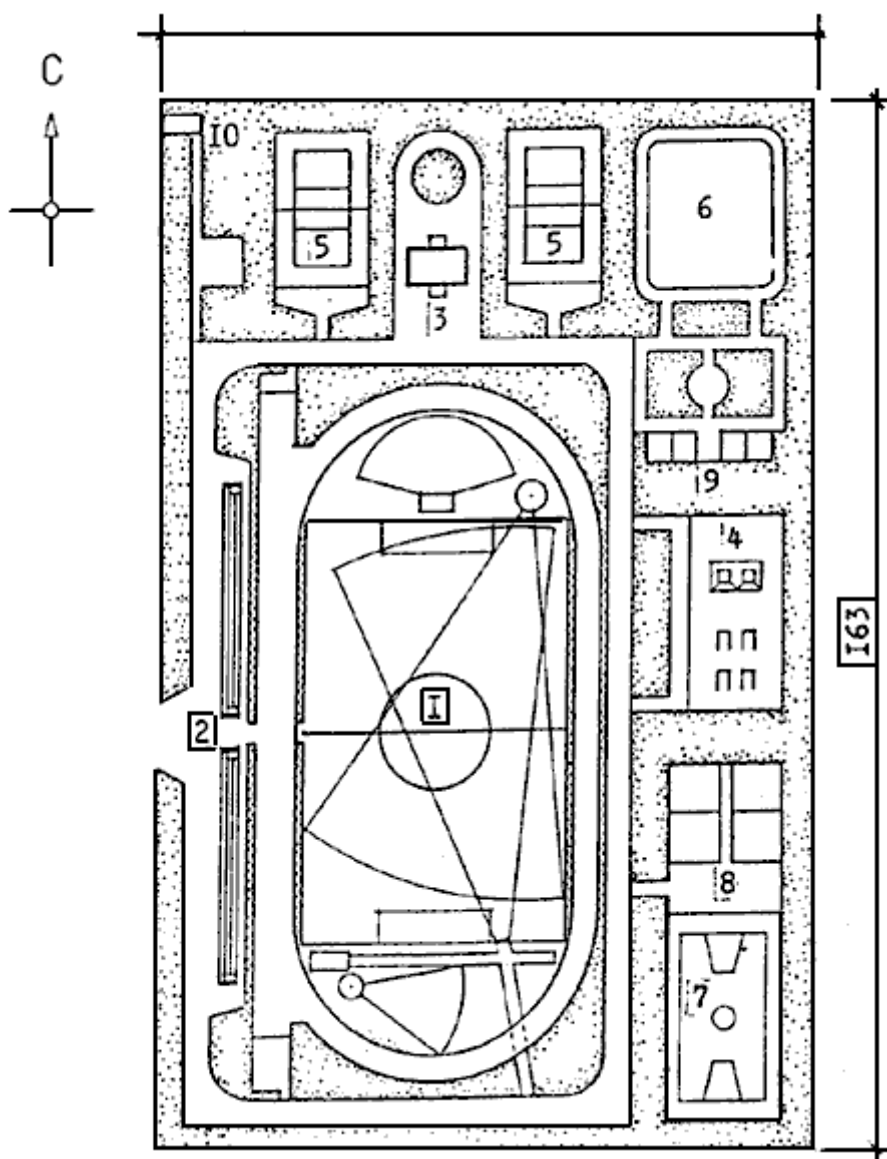
Рис.2. Комплекс спортивных площадок для военного городка на 1000 человек (примерное размещение спортивных сооружений):
