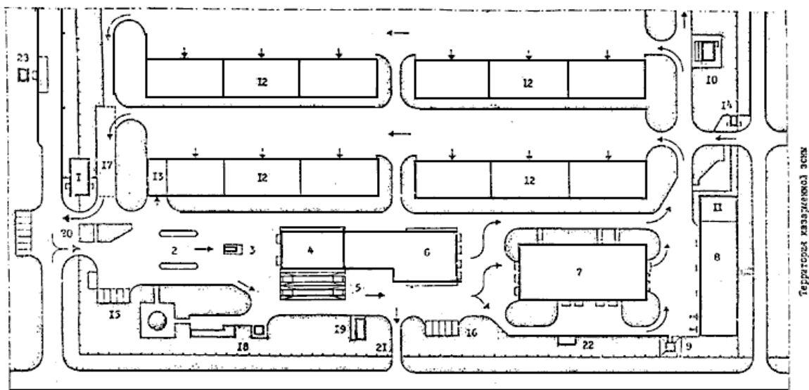
Рис.3. Примерная схема технологической линии парка техники и вооружения (ТВ):
