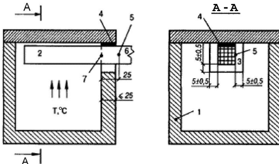
Рисунок Д.3 - Схема встановлення зразка вертикальної стрижневої конструкції на випробувальну піч
