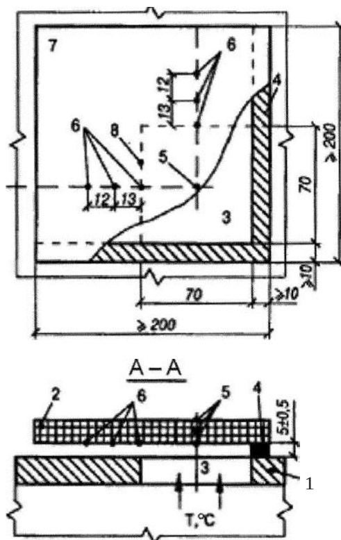
Рисунок Д.1 - Схема встановлення зразка вертикальної огорожувальної конструкції на випробувальну піч
