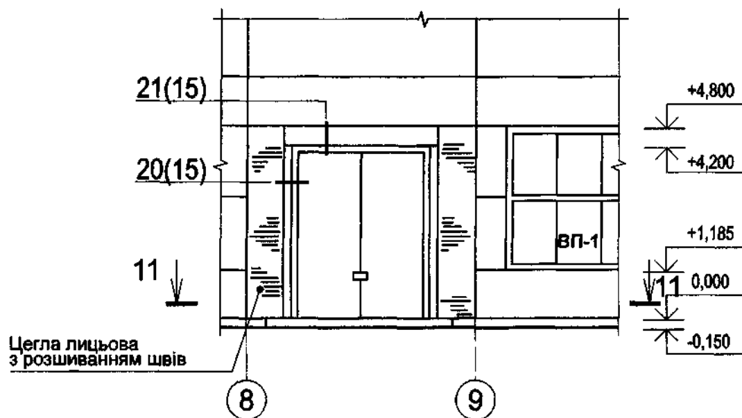
Фрагмент фасаду №3
