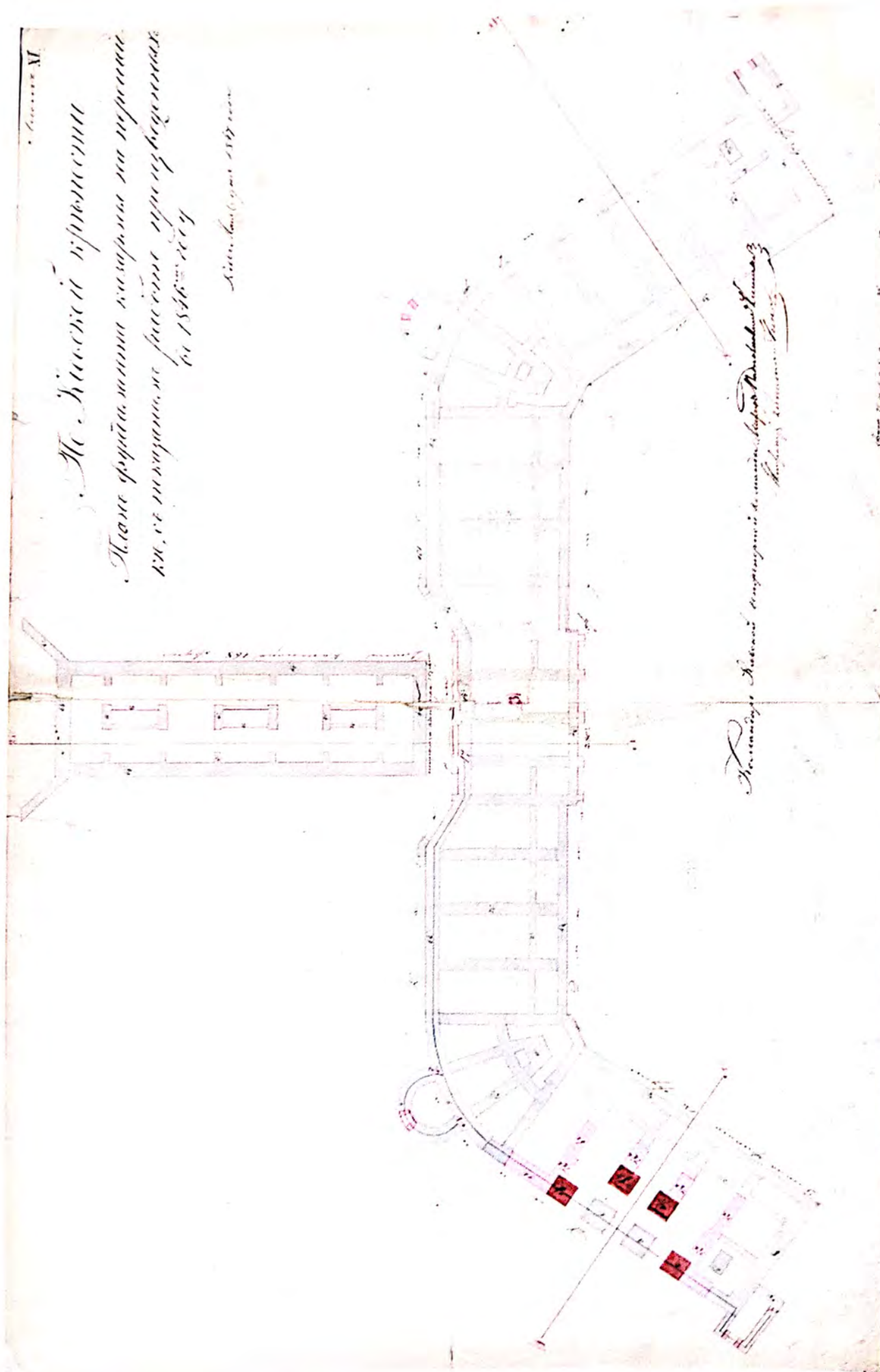
Ил. 2.12. «План фундаментов казарм на перешейке с показанием работ, произведенных в 1846 году». — ЦДІАКУ, ф. 1434, оп. 1, спр. 31, арк. 8.
