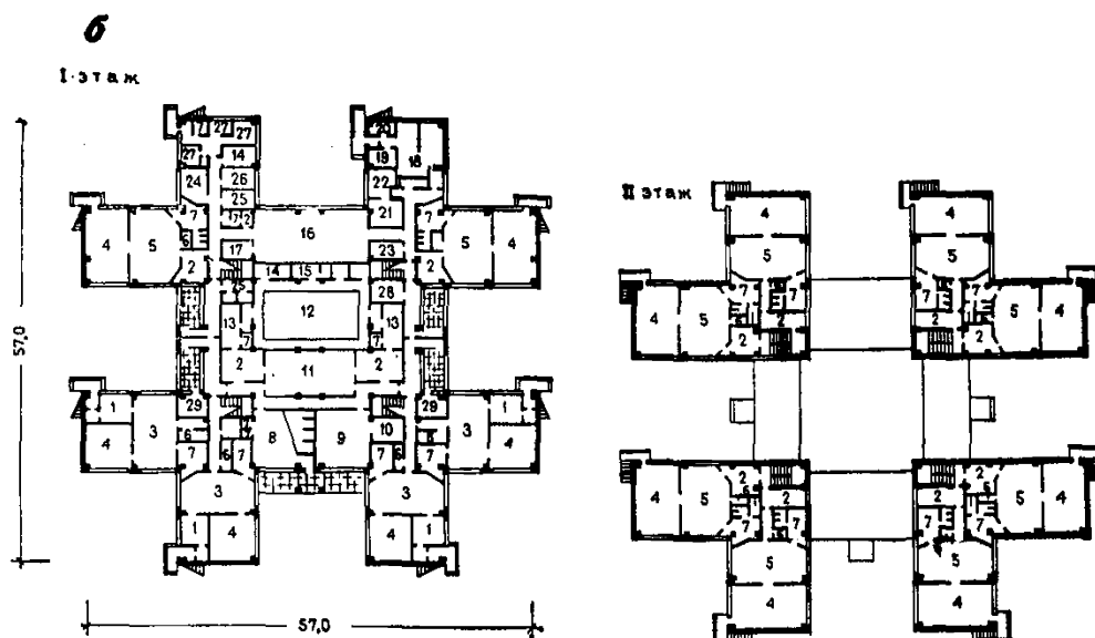
Рис. 37. Экспериментальный проект базового яслей-сада на 330 мест (шифр 76-008)
