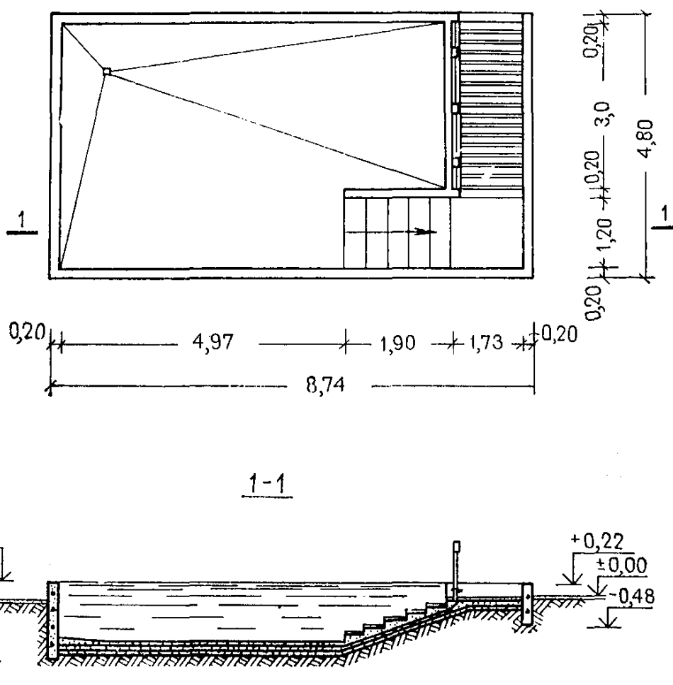
Рис. 9. Пример решения плавательного бассейна
