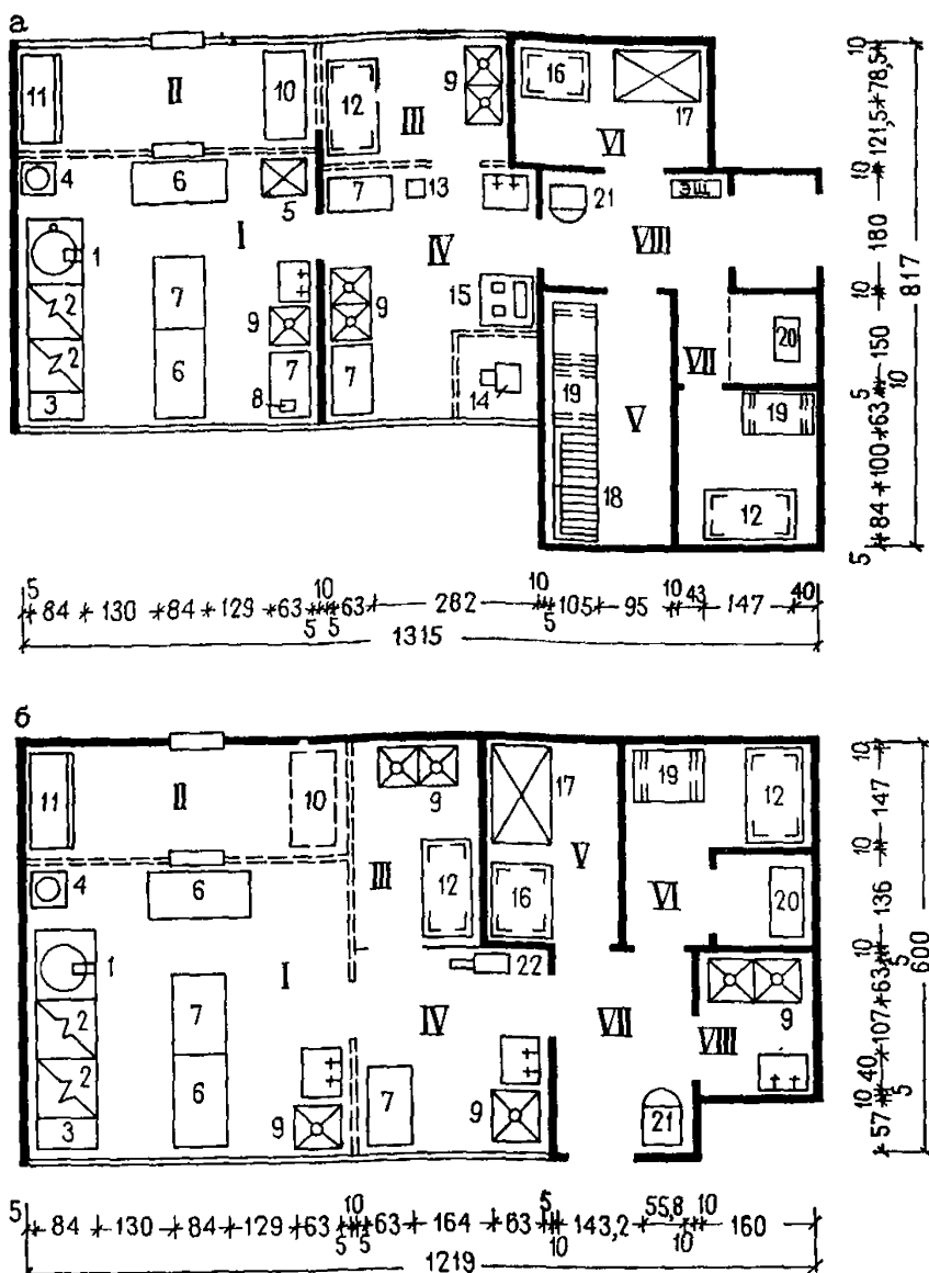
Рис. 31. Функционально-технологическая схема пищеблока яслей-сада на 320 мест
