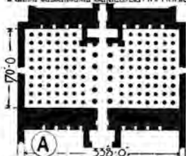
А Многоколонный зал с карнами
