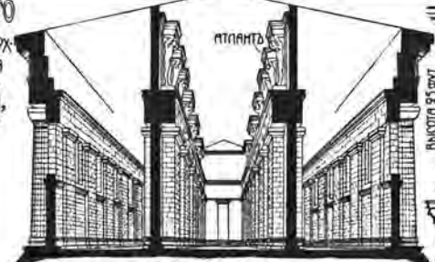
Н РАЗРѢЗЪ
