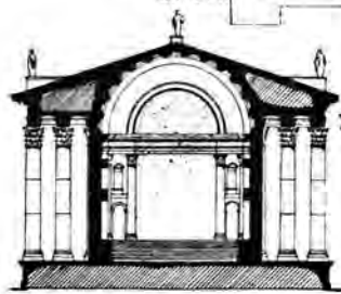
Д РАЗРѢЗЪ БОЛЬШОГО ХРАМА.
