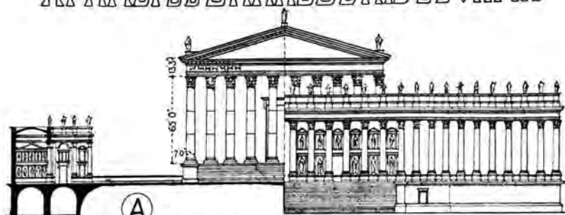
А ПОЛ-РАЗРѢЗЪ ПО Х-Х.
