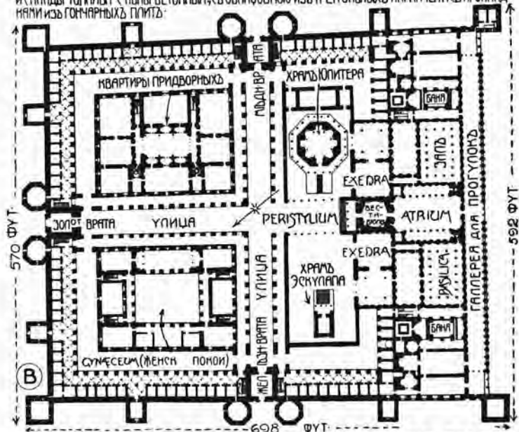
РЕСТАВРИРОВАННЫЙ ПЛАНЪ ДВОРЦА ДИОКЛЕЦИАНА въ Спалато.
