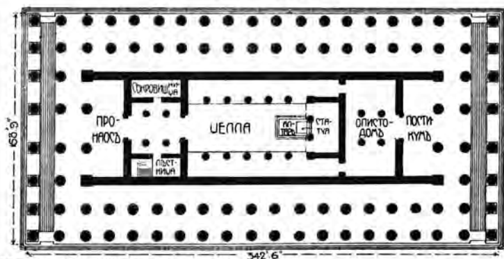
ХРАМЪ АРТЕМИДЫ (ДІАНЫ) В ПИЦЕВѢ
