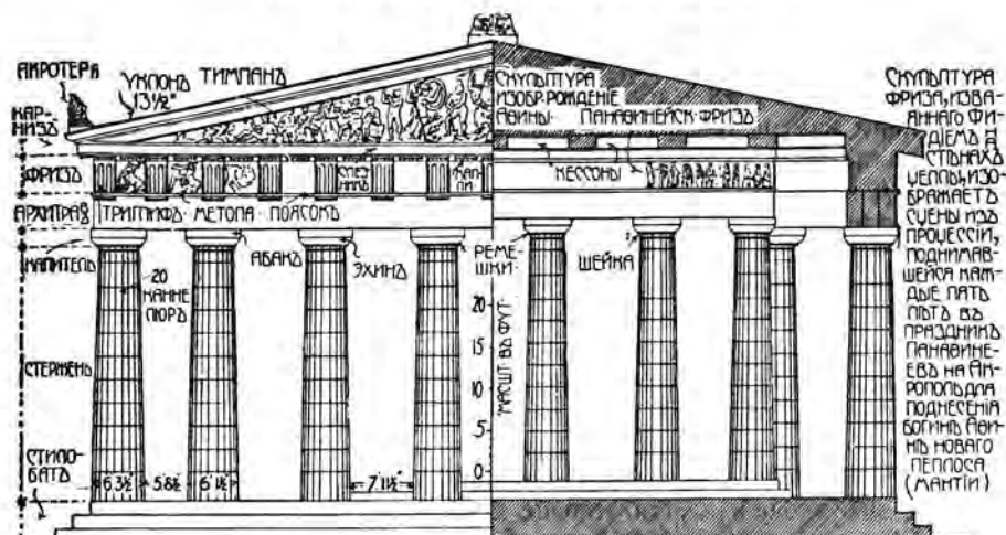
ПОЛОВИНА ВОСТОЧНОГО ФАСАДА ПАРООНОНА.
