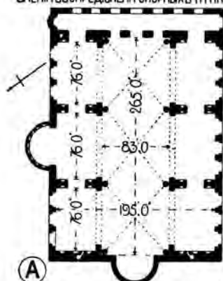
Планъ базилики Константина или Константина. 312 г. по Р.Х.
