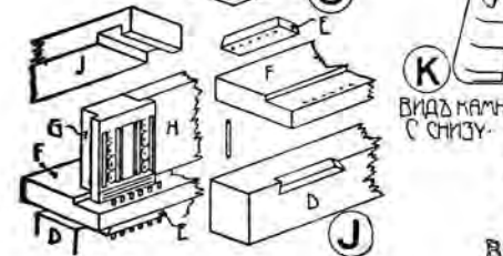
ВОЗСТАНОВЛЕНИЕ ДОРИЧЕСКОГО АНТАБЛЕМЕНТА (ПО ПЕРРО И ШИПЛЕ) И ВОСТАВЛЕНИЕ ЕГО ЧАСТИ ВО РАЗОБЩЕННОМ ВИДЕ.
