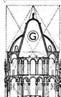
БАПТИСТЕРІА ВЪ ПИЗЪ
