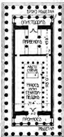
(H) ПЛАНЪ (ПО МѢРКАМЪ)
